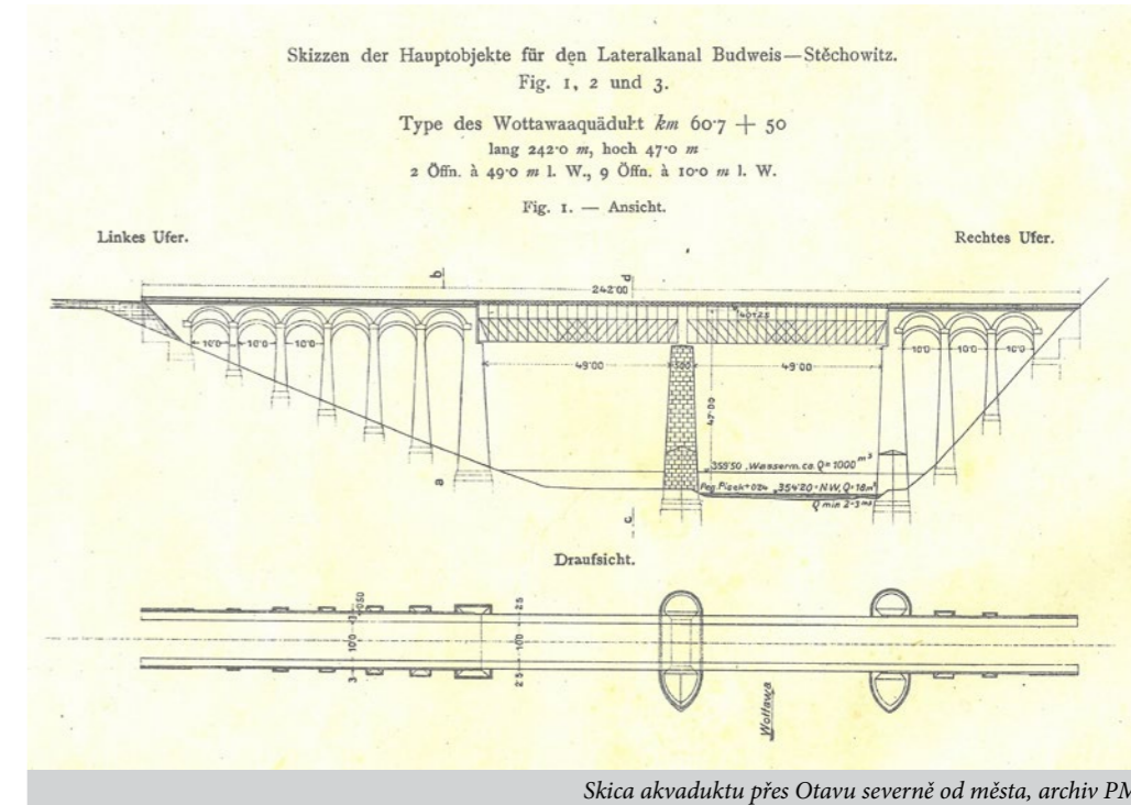
Skica akvaduktu přes Otavu severně od města, archiv PM
